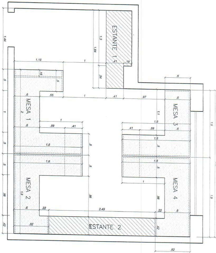
○ CORTE MESAS (4 UNIDADES) ESCALA 1/25 MESAS (verificação abertas no tombo do tempo)
